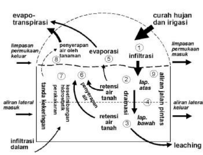
Gambar 2. Bagian-bagian dari kesetimbangan air dalam model WaNuLCAS (1) Infiltrasi, (2,3,4) Redistribusi air dan larutan dalam profil tanah, pengisian kembali air tanah (2) dan drainasi atau pencucian kelebihan air dari dasar profil tanah, (5) Evaporasi tanah, (6) Penyerapan air oleh akar pohon dan tanaman semusim, (7) Kesetimbangan hidraulik melalui akar pohon, (8). Tanda ( signal ) kekeringan yang mempengaruhi pembagian air ke batang/akar, (9) Aliran larutan lewat jalan pintas ( bypass flow )
